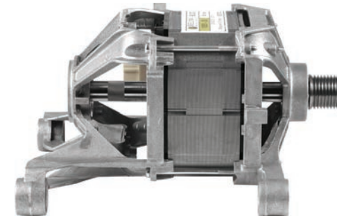
BLDC Motor
