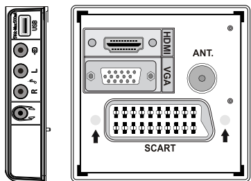
Entrées audio du téléviseur
